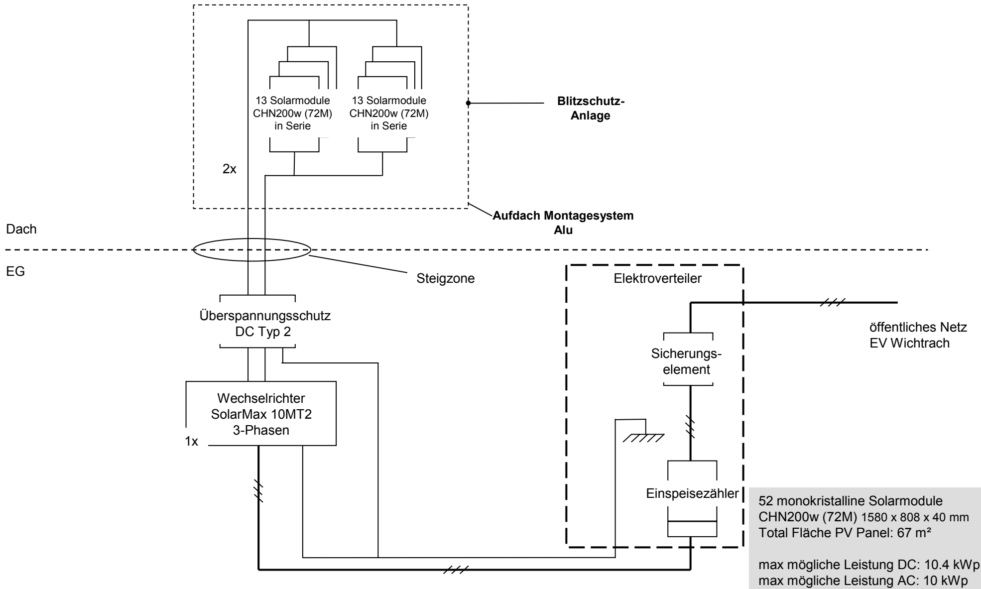
Prinzipschema Photovoltaik Anlage Herrlichkeit 9, 3114 Wichtrach 03.06.2012 Heinrich Schneeberger Schneeberger Haustechnik, 3114 Wichtrach
