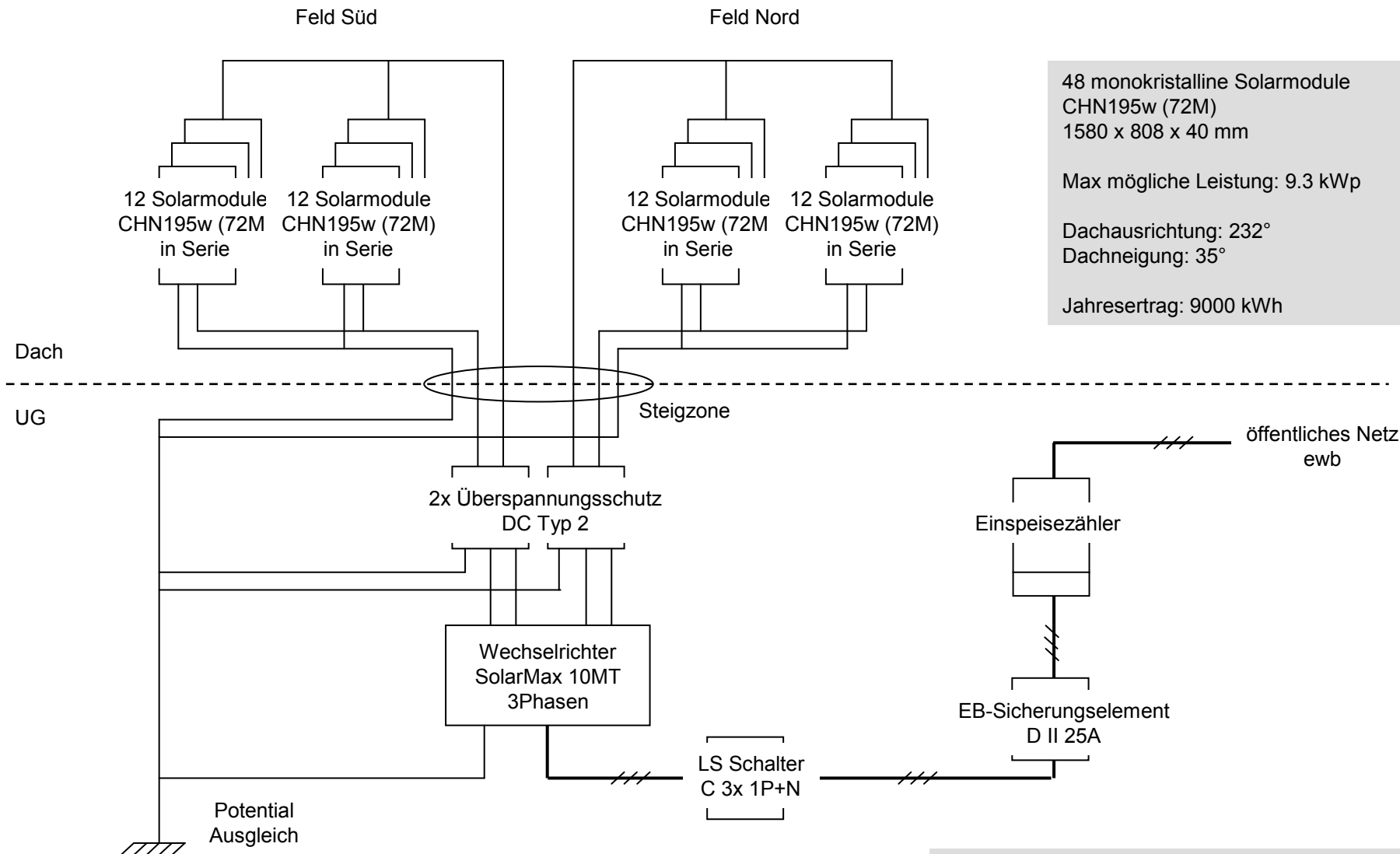
Prinzipschema Photovoltaik Anlage Sagerstrasse 4, 3006 Bern 10.08.2011 Heinrich Schneeberger Schneeberger Haustechnik, Wichtrach
